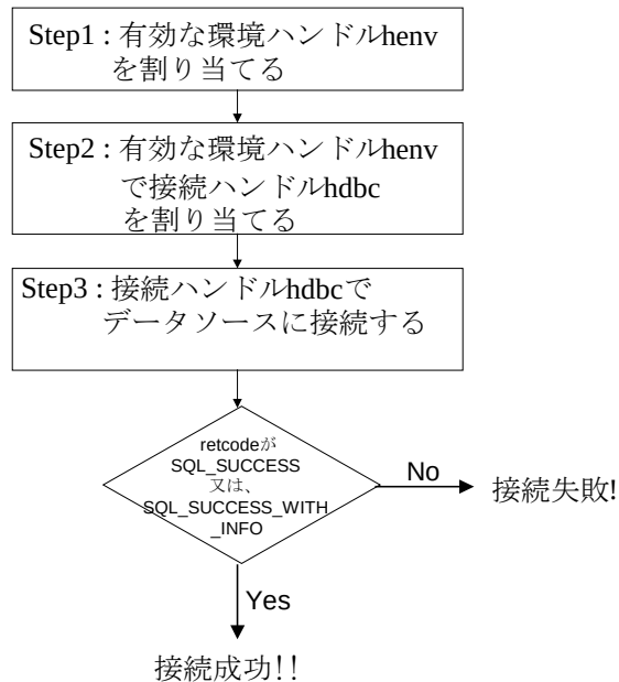
図 3-2: データソースへの接続のためのプログラム・フロー
