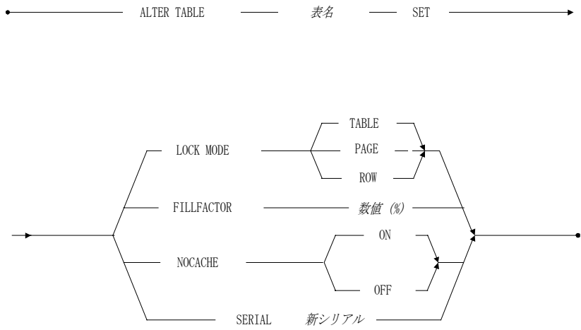
図 2-1：構文ダイアグラムの簡単な例
