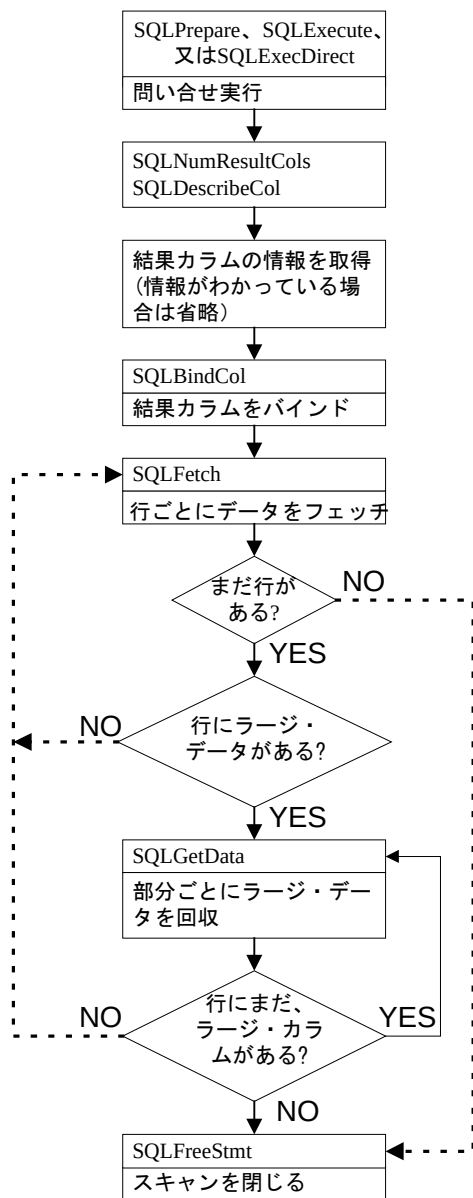
図 5-1: データベースからデータを回収するためのプログラム・フロー
