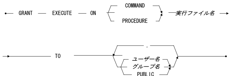
図 12-8 GRANT EXECUTE 文の構文
