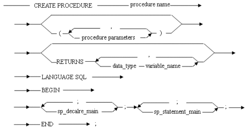
図 12-5 SQL ストアド・プロシージャを作成する構文
