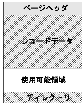
図 5-3: データページのフォーマット
