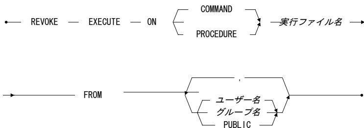
図 12-9 REVOKE EXECUTE 文の構文
