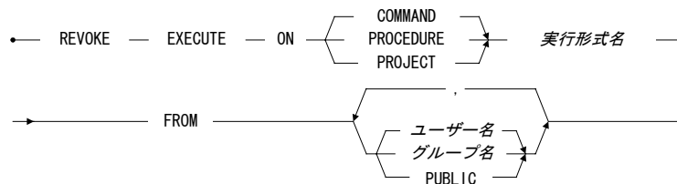
図 11-5 REVOKE EXECUTE 権限の構文
