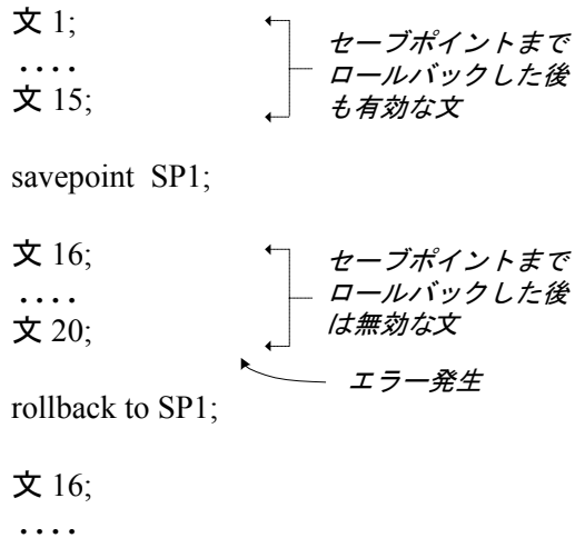
図 9-2: セーブポイントの使用法
