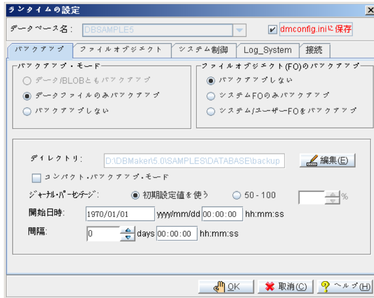
図25-1 ランタイム設定の「バックアップ」のページ
