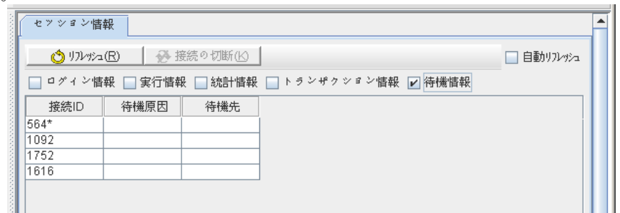
図 24-5 セッション情報:待機情報
