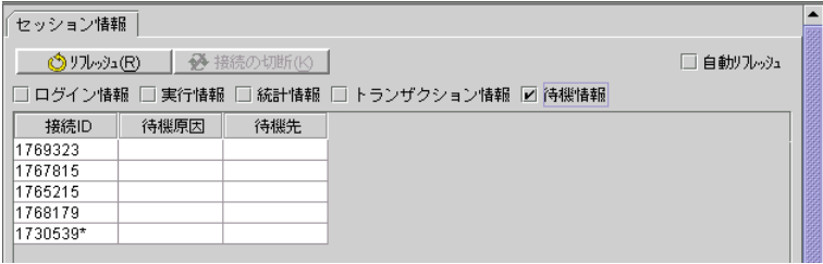
図 24-5 セッション情報:待機情報
