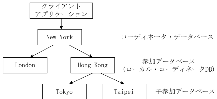
図15-3: DBMaster の分散構造
