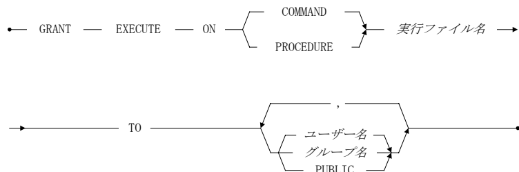
図 12-6 GRANT EXECUTE 文の構文
