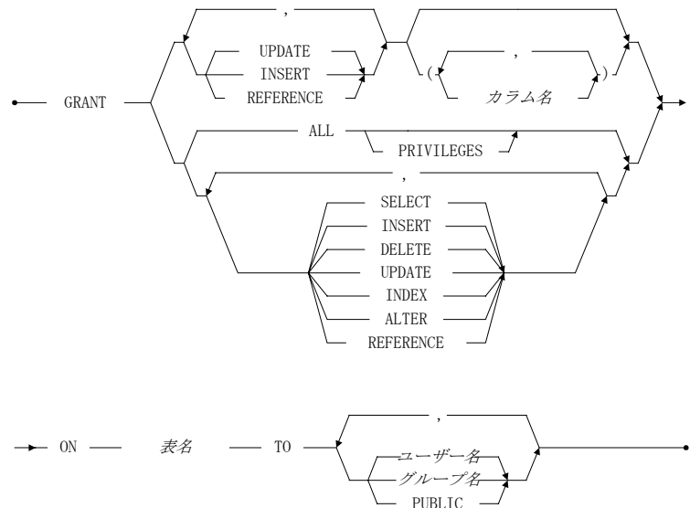
図8-11 GRANT(オブジェクト権限)文の構文
