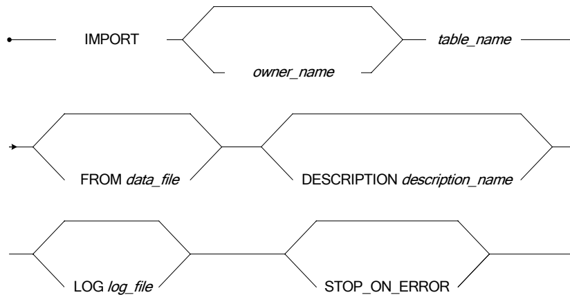
図 6-1 IMPORT構文
