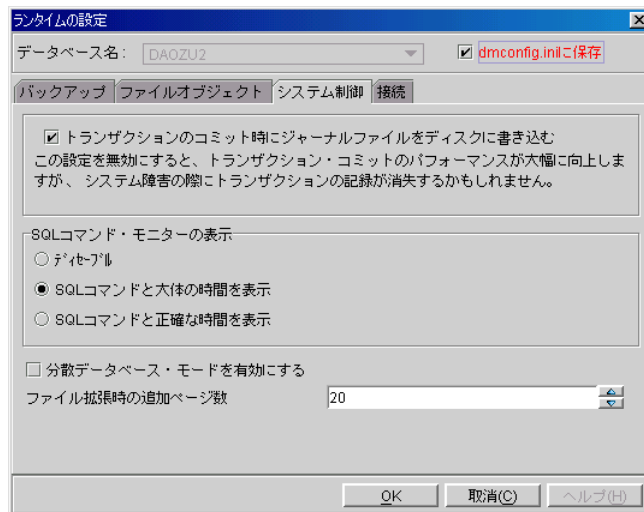
図 24-3 ランタイム設定の [システム制御] のページ
