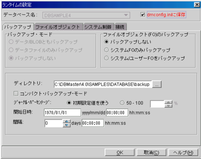
図 24-1 ランタイム設定の [バックアップ] のページ
