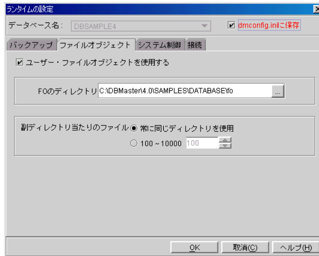
図 24-2 ランタイム設定の [ファイルオブジェクト] のページ
