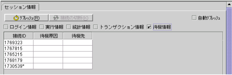
図 23-5 セッション情報:待機情報
