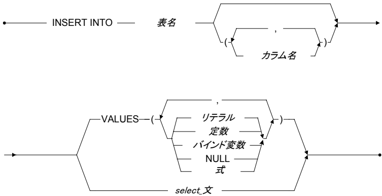
図 6-1: INSERT 文の構文
