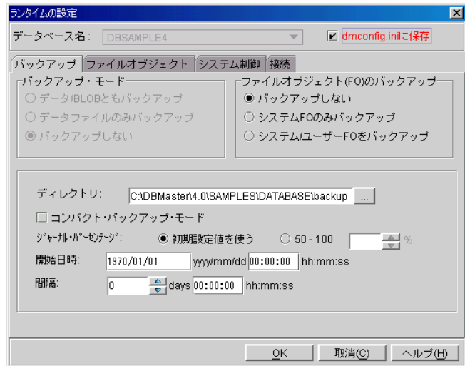
図 22-1 ランタイム設定の [バックアップ] のページ
