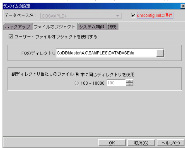
図 22-2 ランタイム設定の「ファイルオブジェクト」のページ
